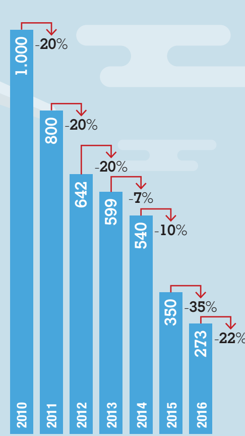
FIGURA 4. EVOLUZIONE DEL PREZZO DELLE BATTERIE AL LITIO ($/kWh)
