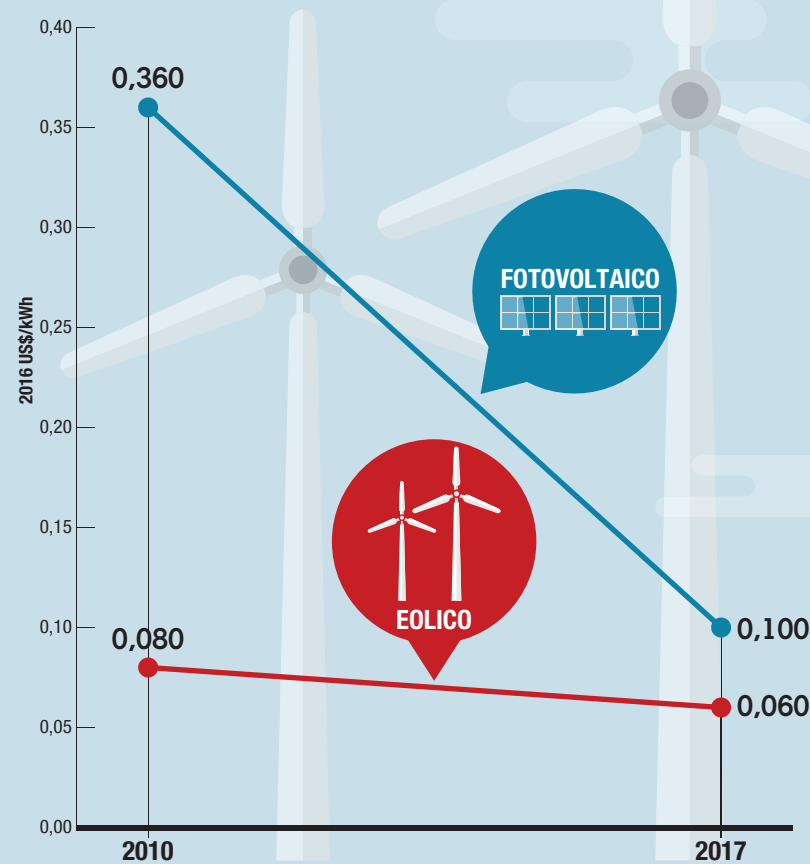
FIGURA 3. EVOLUZIONE DEL COSTO DI GENERAZIONE DEL KWH DA IMPIANTI FOTOVOLTAICI ED EOLICI “UTILITY SCALE” (media mondiale ponderata)
