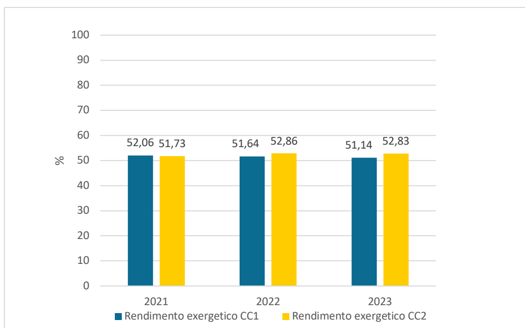
Figura 17 - Rendimento exergetico
