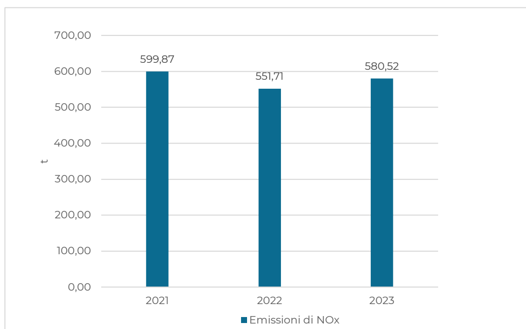
Figura 6 - Emissioni in atmosfera di NO x : quantità
