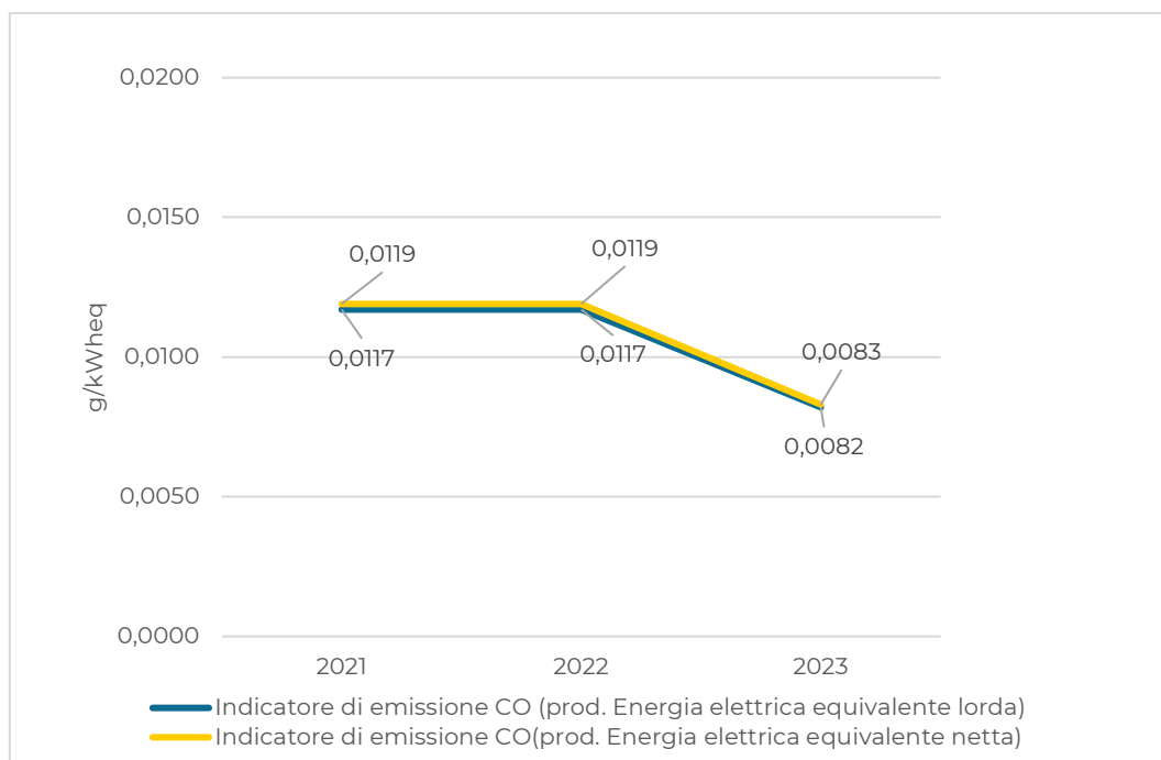
Figura 9 - Emissioni in atmosfera di CO: indicatori di emissione
