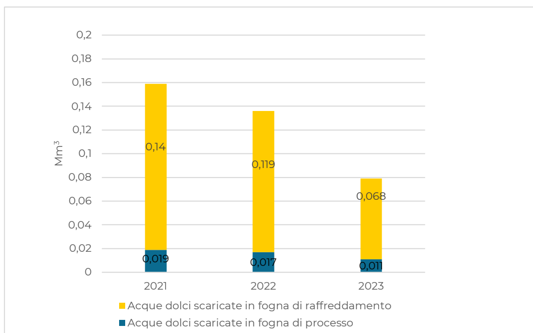
Figura 14 - Scarichi idrici
