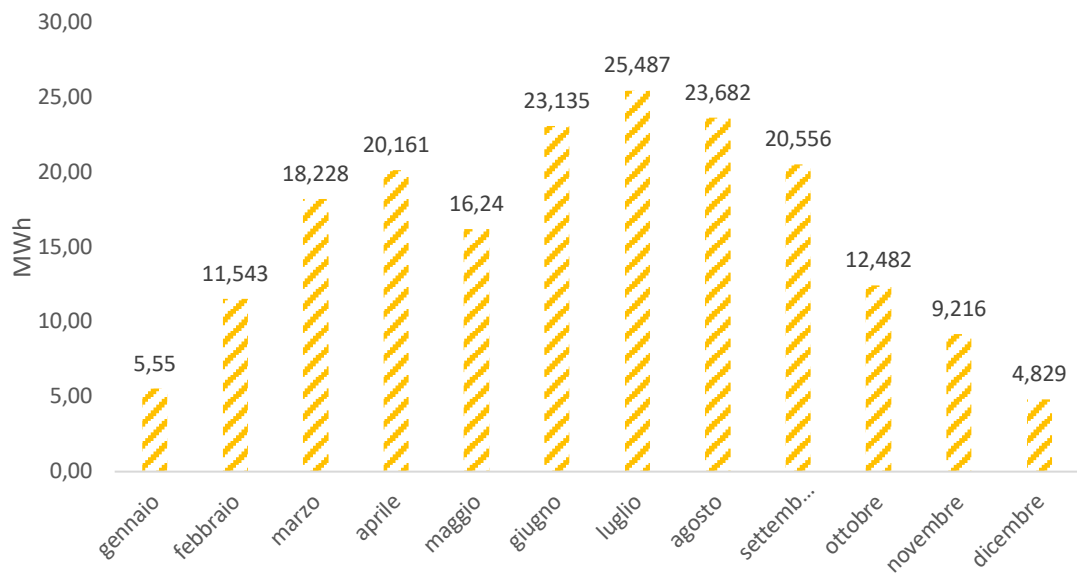
Figura 20 - Energia elettrica prodotta nel 2023
