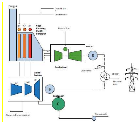
Figura 4 - Schema di processo di un ciclo combinato
