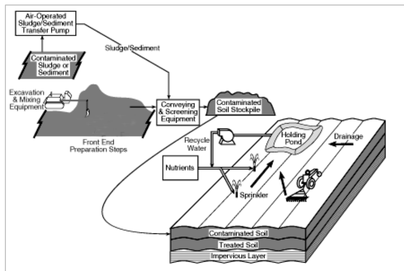
Figura 6-20 Schema Biopile (fonte: FRTR, EPA)
