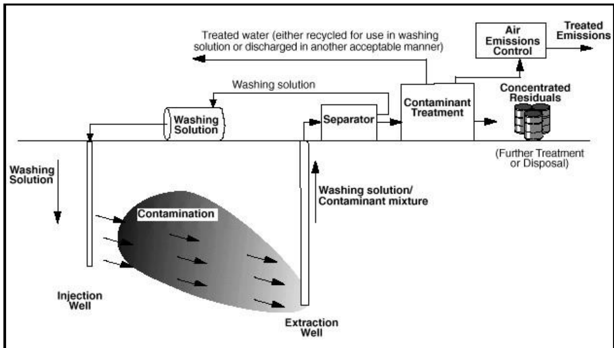
Figura 6-14 Schema del Soil Flushing (fonte: EPA,1996)
