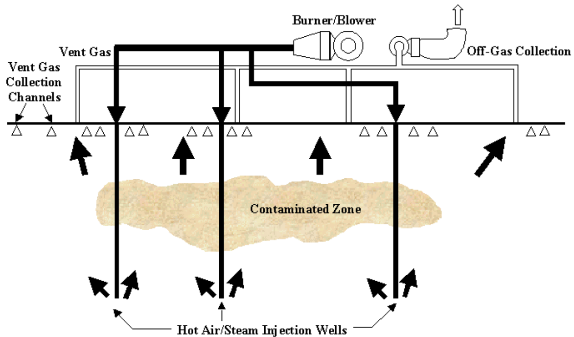
Figura 6-31 Schema di Trattamento termico in situ (Fonte: FRTR, EPA)
