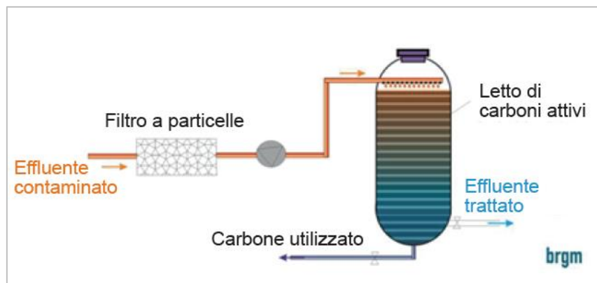
Figura 6-27 Schema Adsorbimento (Fonte: Quelles techniques pour quels traitements - Analyse couts-benefices Rapport Final, BRGM, 2010©BRGM/RP-58609-FR - modificato)
