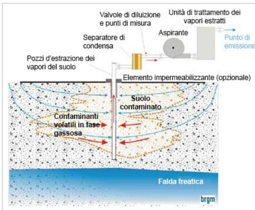
Figura 6-16 Schema di SVE (Fonte: Quelles techniques pour quels traitements - Analyse coûts-bénéfices Rapport Final, BRGM, 2010 ©BRGM/RP-58609-FR - modificata)
