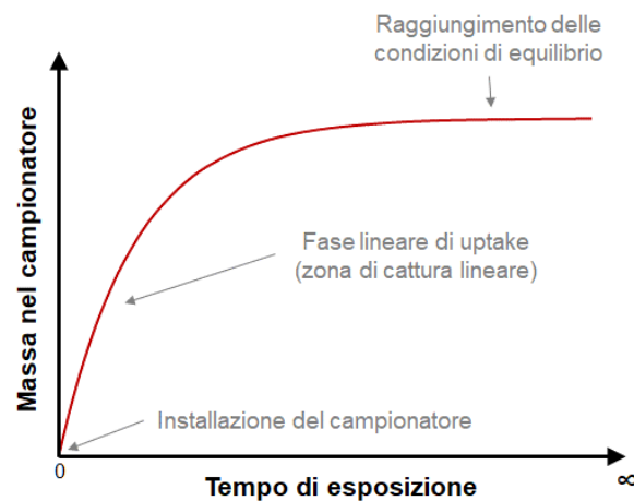
Figura 8-7: Massa di contaminante adsorbita nel campionatore passivo in funzione del tempo di esposizione.
