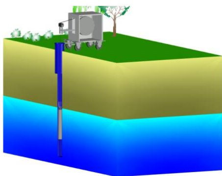
Figura 8-2: Il dispositivo e-hyrec® posizionato in falda. È costituito dalla parte calata in pozzo e dal sistema di movimentazione, gestione e controllo posto a bocca pozzo.
