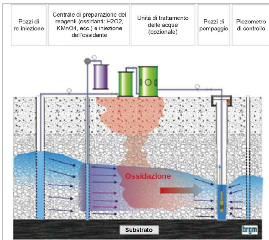
Figura 6-13 Schema Ossidazione chimica (Fonte: Quelles techniques pour quels traitements - Analyse coûts-benefices Rapport Final, BRGM, 2010 ©BRGM/RP-58609-FR – modificata)
