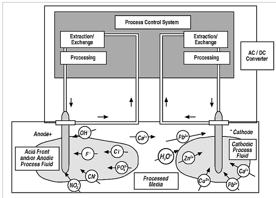
Figura 6-9 Schema dell'Elettrocinesi (Fonte: FRTR, EPA)
