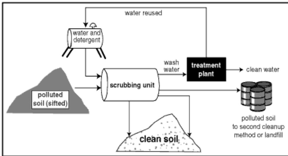
Figura 6-15 Schema del Soil Washing (fonte: EPA)
