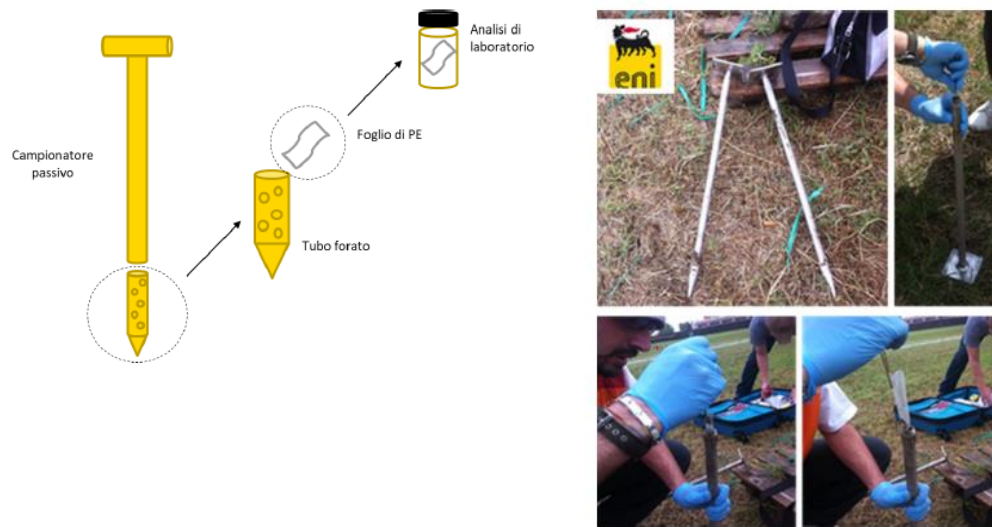
Figura 8-10: Campionatore passivo per monitoraggio superficiale – applicazione manuale
