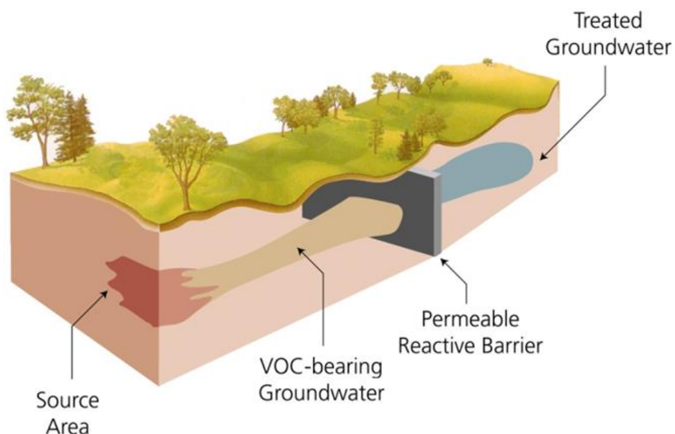
Figura 6-7 Funzionamento della barriera continua (fonte: Professor Petrangeli Papini)
