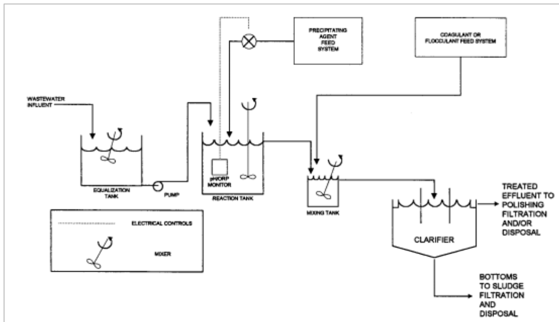
Figura 6-25 Schema della Chiariflocculazione (Fonte: FRTR, EPA)
