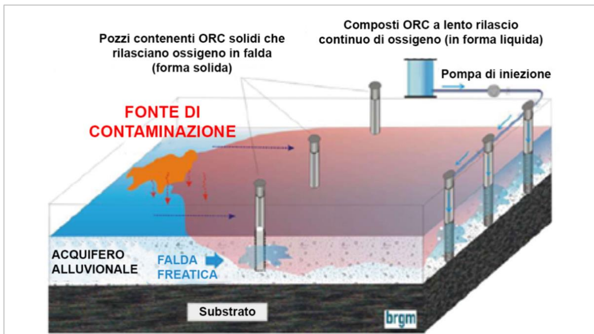
Figura 6-1 Schema del principio di biodegradazione in situ (Fonte: Quelles techniques pour quels traitements - Analyse coûts-benefices Rapport Final, BRGM, 2010 ©BRGM/RP-58609-FR - modificato)
