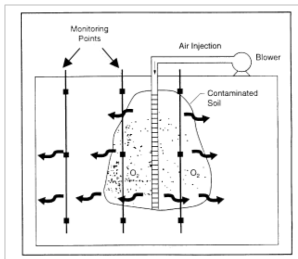
Figura 6-17 Schema di funzionamento del BV (fonte: AFCEE, 1994 / USACE 2002)
