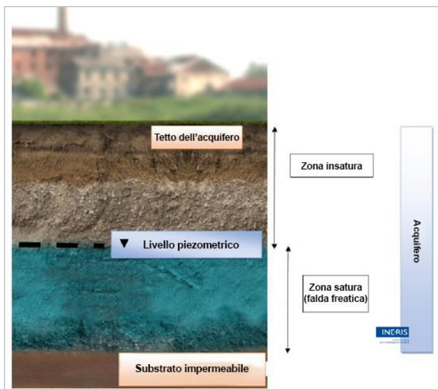
Figura 1-1 Schema di Sistema suolo-sottosuolo – falda libera (Fonte: Guide méthodologique relatif au Plan de Conception des Travaux (PCT), INERIS 2019 - modificato)
