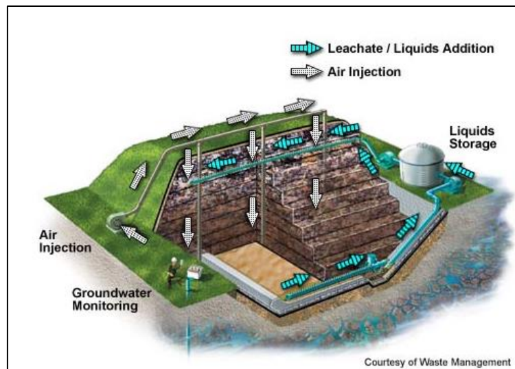
Figura 6-22 Schema di bioreattore (EPA-Waste Management)
