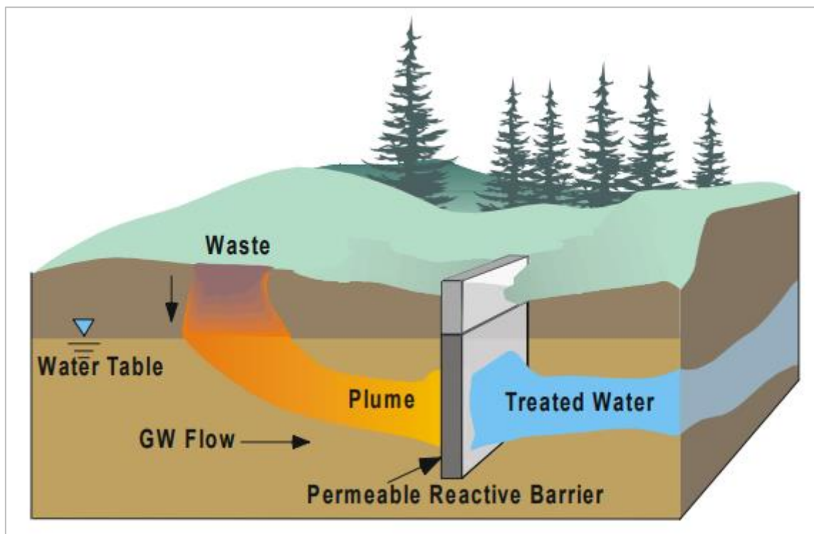
Figura 6-6 Schema delle Barriere Reattive Permeabili (fonte: EPA, 1998)
