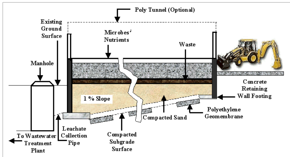
Figura 6-19 Schema di funzionamento del Landfarming (fonte: FRTR, EPA)
