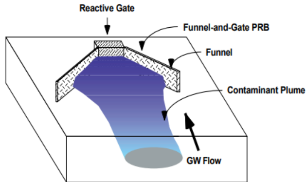
Figura 6-8 Funzionamento del Funnel and Gate (fonte: EPA, 1998)
