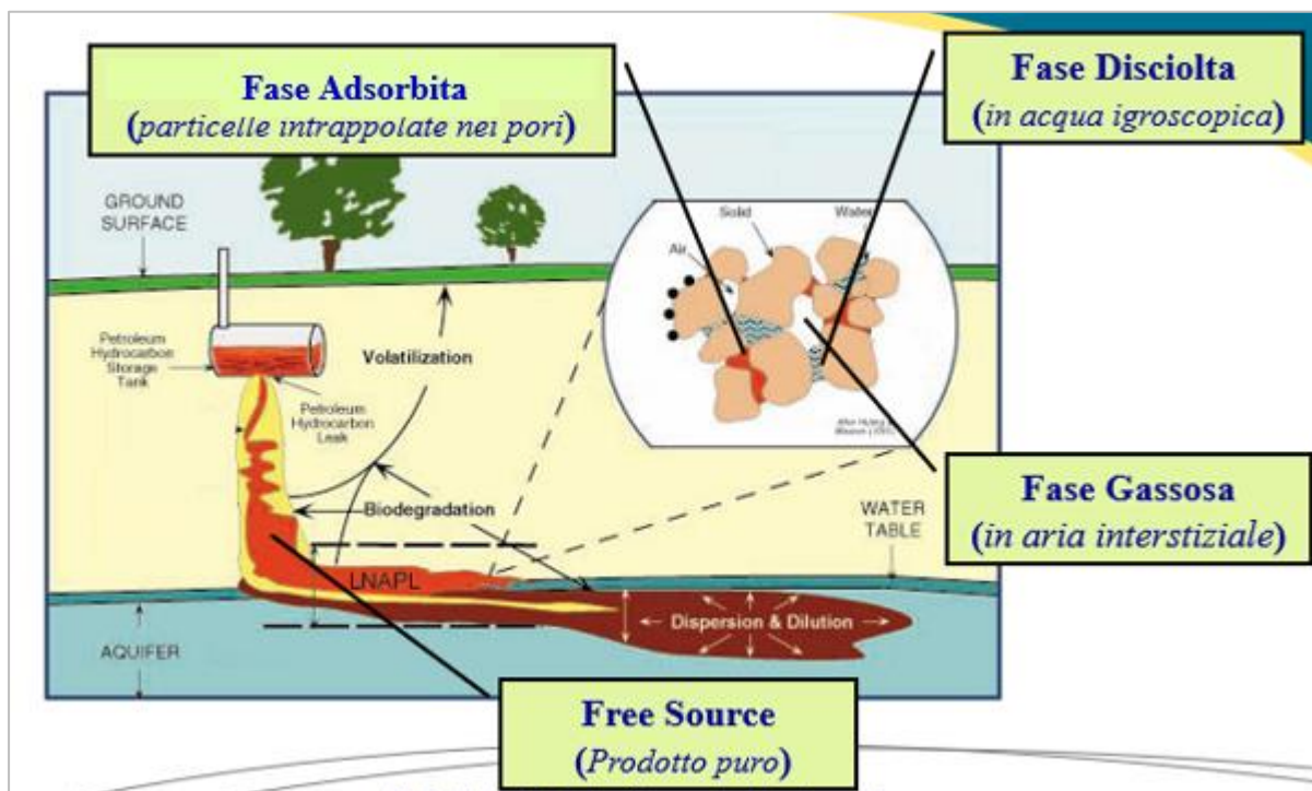
Figura 1-3 Schema delle fasi del sottosuolo (Fonte: Tecnologie per la bonifica di siti contaminati: fondamenti teorici ed applicazioni, MWH, 2014-modificata)
