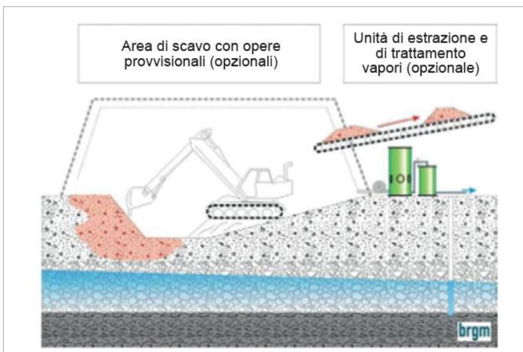
Figura 6-23 Schema di scavo e smaltimento (Fonte: Quelles techniques pour quels traitements - Analyse coûts-benefices Rapport Final, BRGM, 2010©BRGM/RP-58609-FR - modificato)
