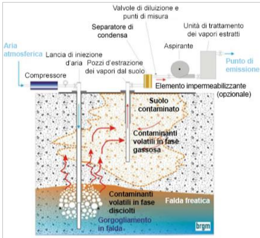
Figura 6-4 Schema di funzionamento AS- SVE (Fonte: Quelles techniques pour quels traitements - Analyse coûts-bénéfices Rapport Final, BRGM, 2010 ©BRGM/RP-58609-FR - modificata)
