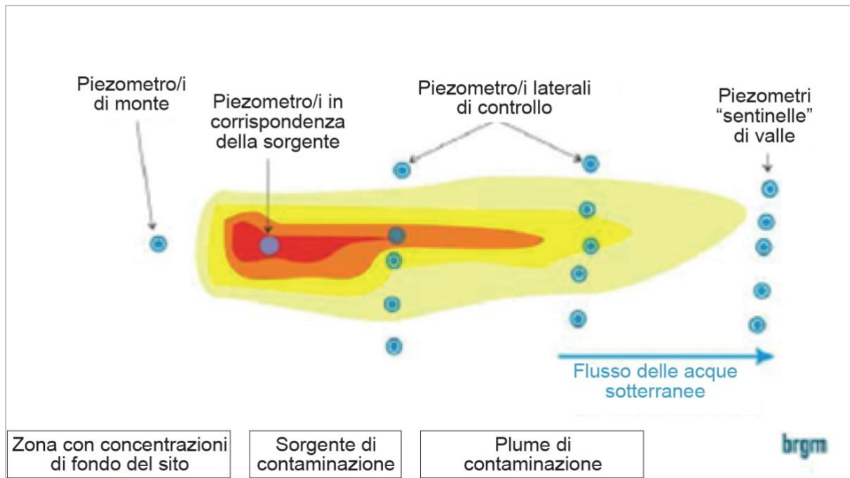
Figura 6-2 Ubicazione dei piezometri di monitoraggio intervento MNA (Fonte: Quelles techniques pour quels traitements - Analyse coûts-bénéfices Rapport Final, BRGM, 2010 ©BRGM/RP-58609-FR - modificata)
