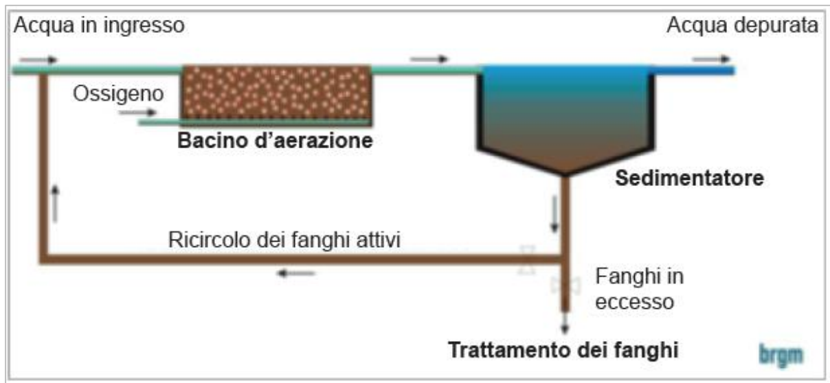
Figura 6-21 Schema della tecnologia a fanghi attivi (Fonte: Quelles techniques pour quels traitements - Analyse coûts-bénéfices Rapport Final, BRGM, 2010 ©BRGM/RP-58609-FR - modificata)
