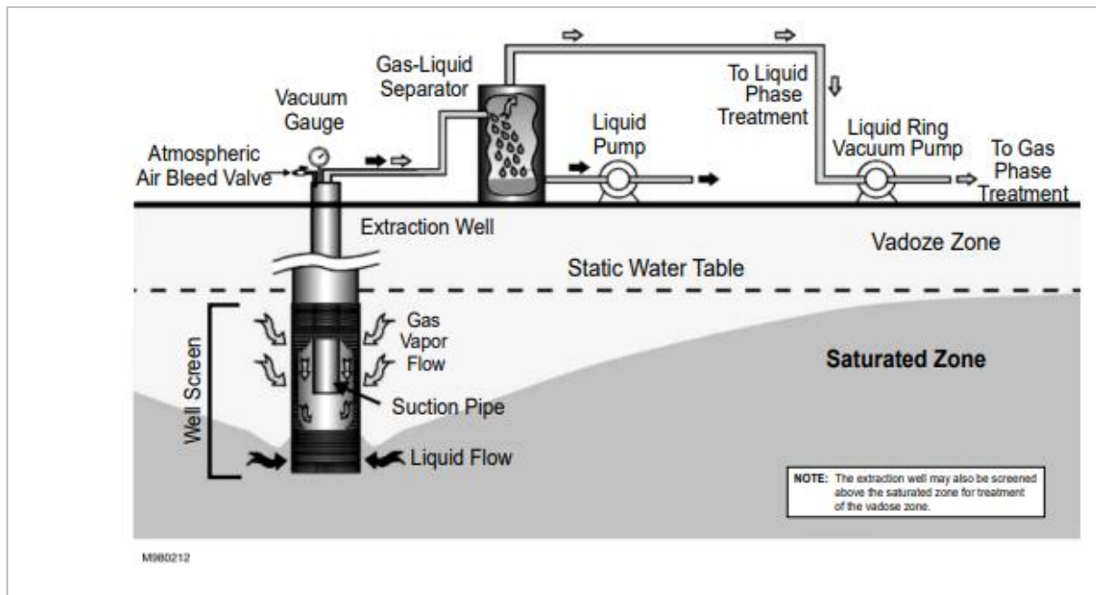
Figura 6-11 Schema del TPE (Fonte: After EPA 1997)
