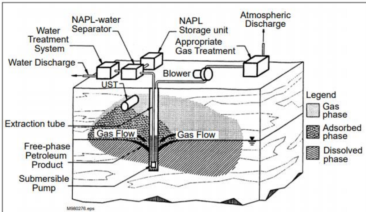
Figura 6-10 Schema della tecnologia DPE (Fonte: After USEPA 1995)
