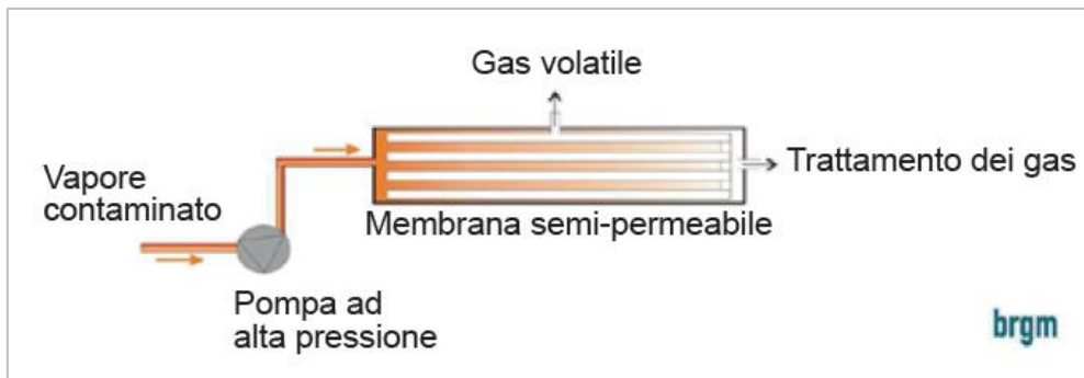
Figura 6-29 Schema Osmosi Inversa (Fonte: Quelles techniques pour quels traitements - Analyse couts-benefices Rapport Final, BRGM, 2010 ©BRGM/RP-58609-FR - modificato)
