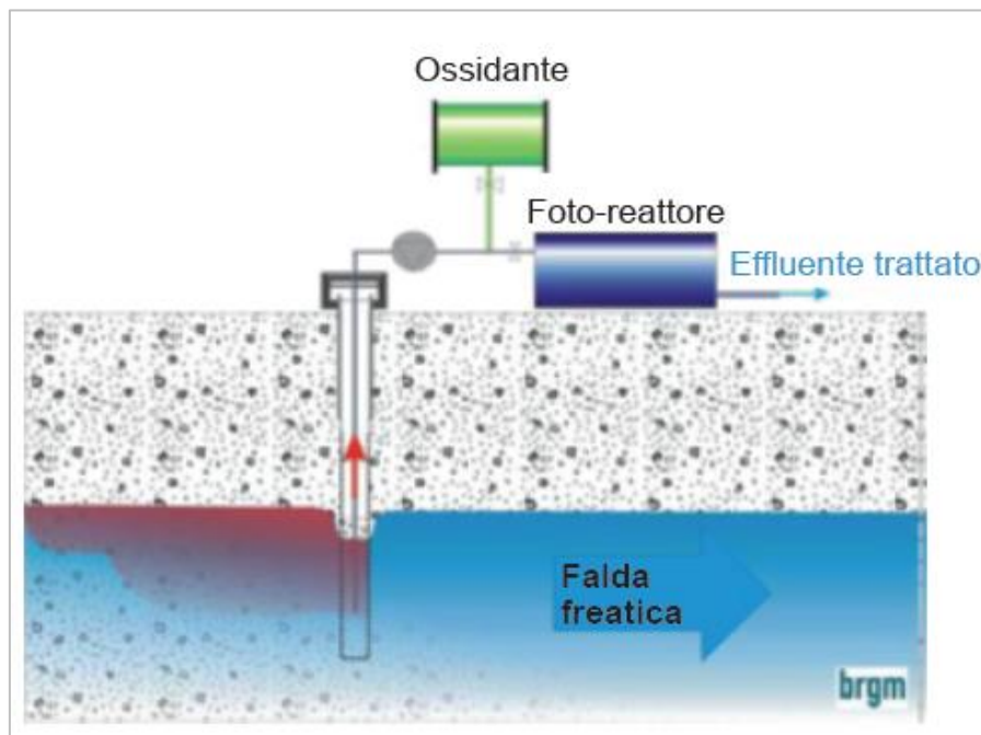
Figura 6-30 Schema Ossidazione UV (Fonte: Quelles techniques pour quels traitements - Analyse couts-benefices Rapport Final, BRGM, 2010 ©BRGM/RP-58609-FR - modificato)
