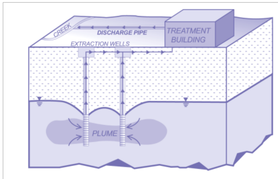
Figura 6-5 Schema di trattamento mediante P&T (fonte: U.S. EPA)
