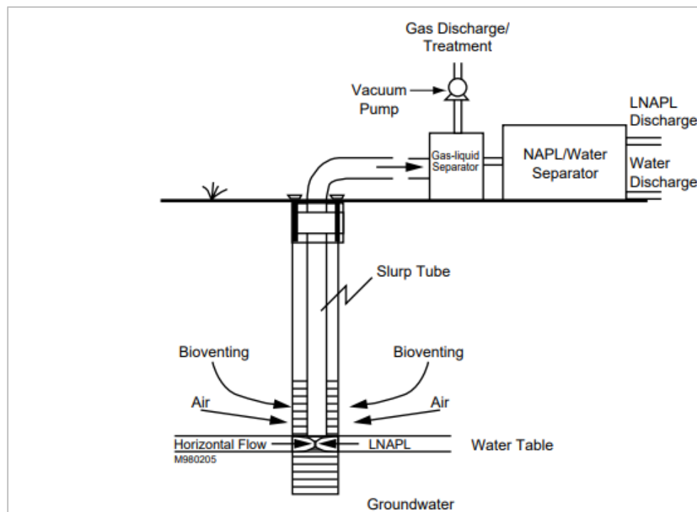
Figura 6-12 Schema del Bioslurping (Fonte: After AFCEE 1994b)
