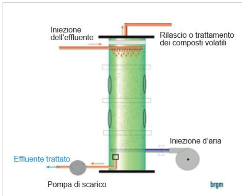
Figura 6-28 Schema Strippaggio (Fonte: Quelles techniques pour quels traitements - Analyse coûts-bénéfices Rapport Final, BRGM, 2010 ©BRGM/RP-58609-FR - modificato)
