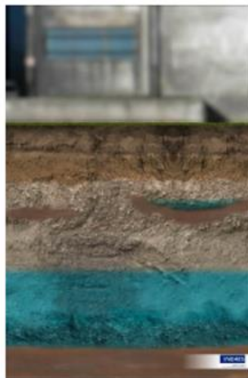
Falda sospesa
