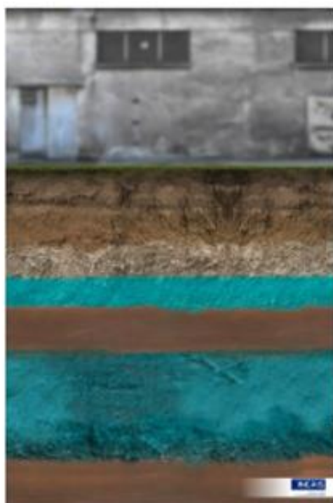
Falda confinata
