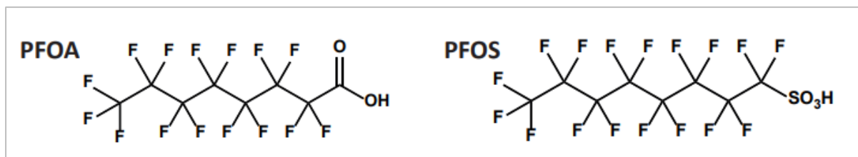
Figura 2-6: Struttura molecolare PFAS
