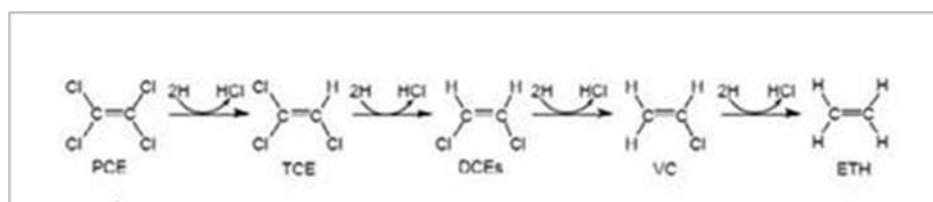
Figura 2-4 Catena di degradazione del Tetracloroetilene
