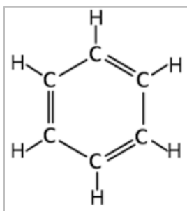
Figura 2-2 Molecola di Benzene
