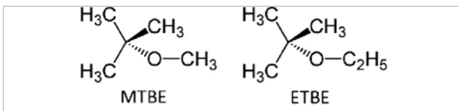
Figura 2-5 Molecole di MTBE e ETBE
