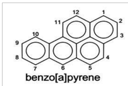
Figura 2-3 Molecola di Benzo(a)pirene
