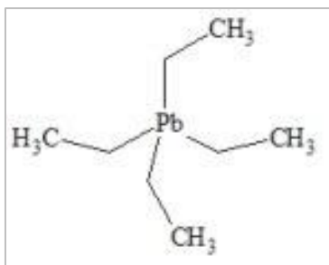
Figura 2-7 Molecola di Piombo Tetraetile
