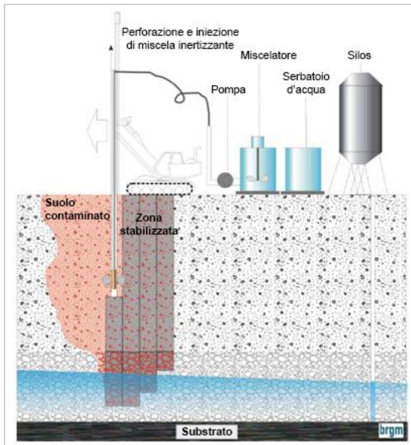
Figura 6-18 Schema di solidificazione e stabilizzazione (Fonte: Quelles techniques pour quels traitements - Analyse coûts-bénéfices Rapport Final, BRGM, 2010 ©BRGM/RP-58609-FR - modificata)
